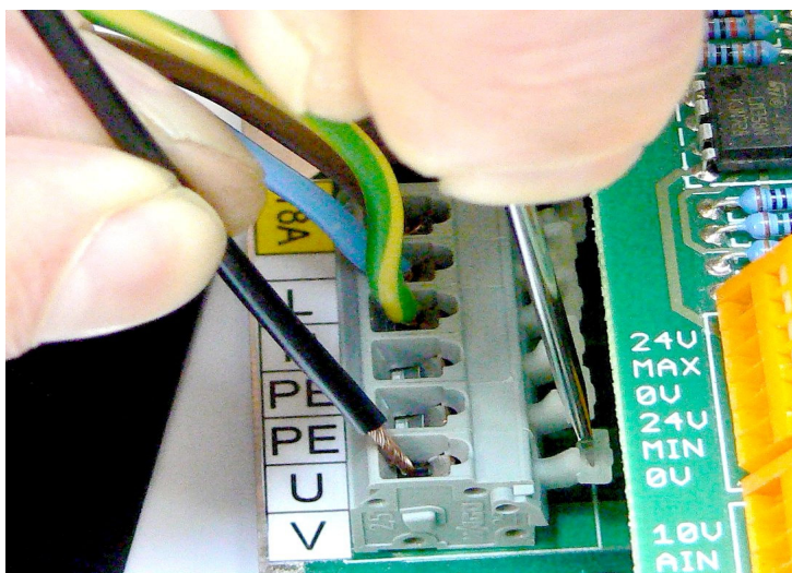
obr. 9 - připojení vodičů
